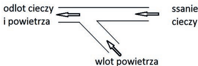
Rys. 6. Zasada działania eżektora.
