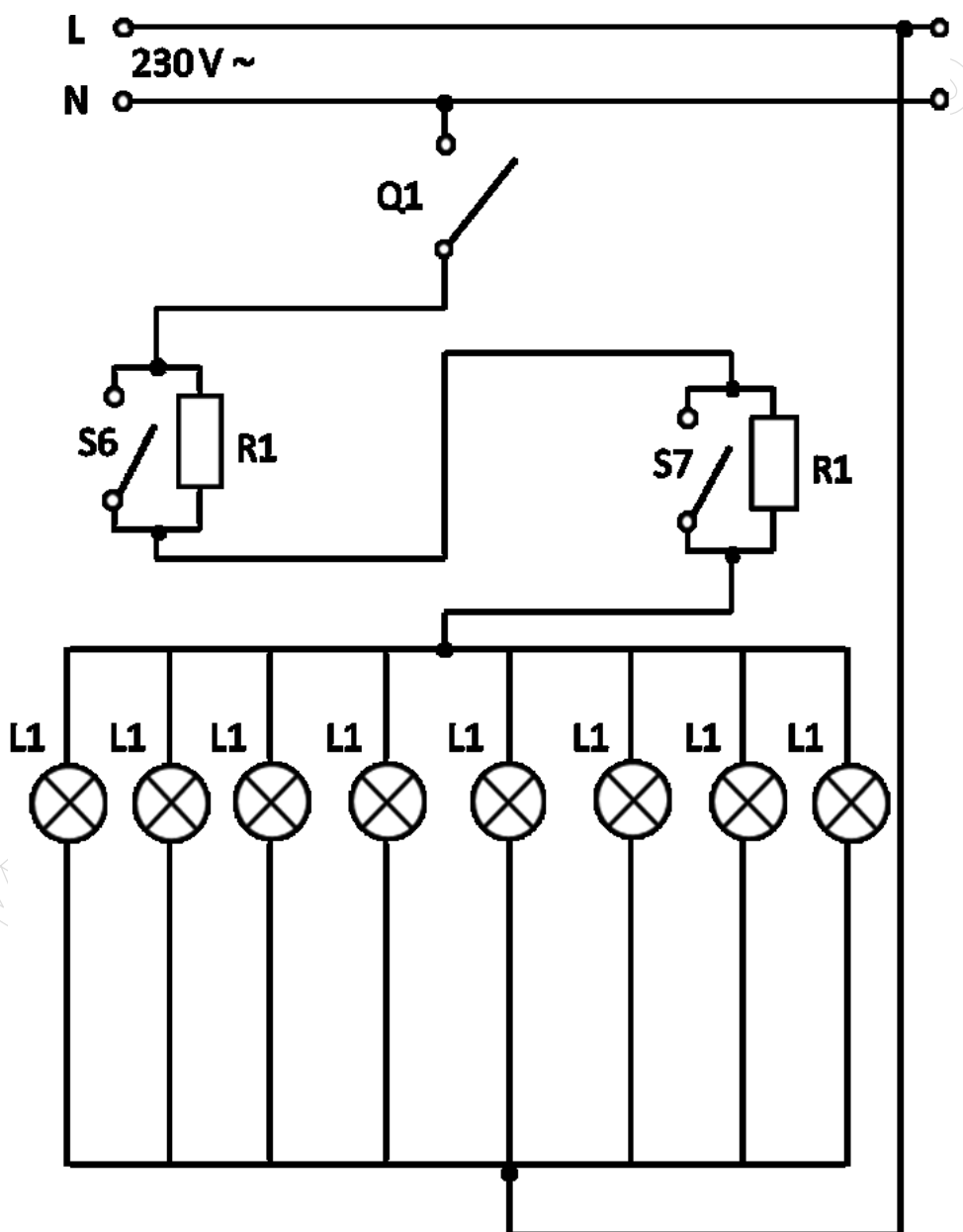
Schemat ideowy układu podświetlenia
