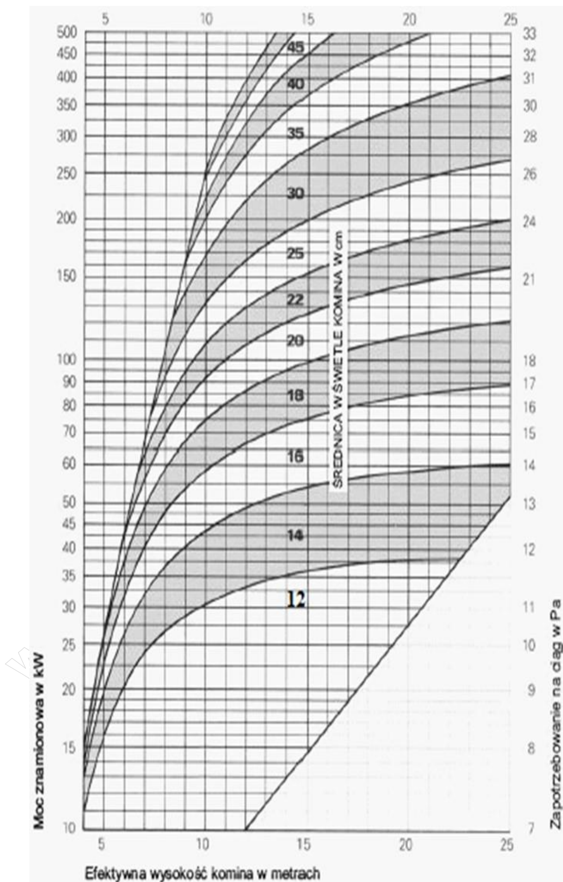
Rysunek 1. Diagramy doboru średnicy komina dla kotła grzewczego na olej opałowy
