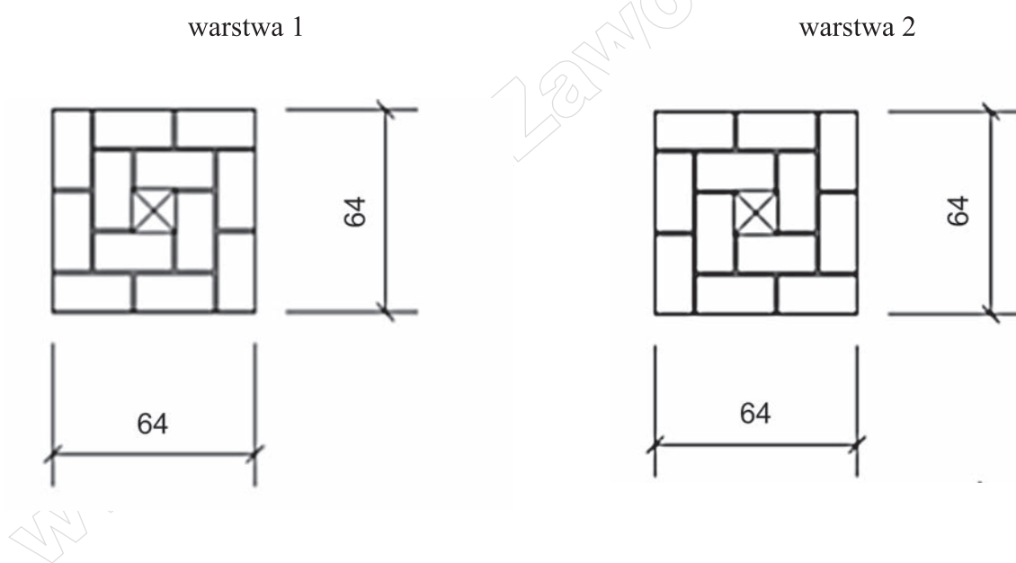
Rysunek 1. Układ cegieł w słupie
