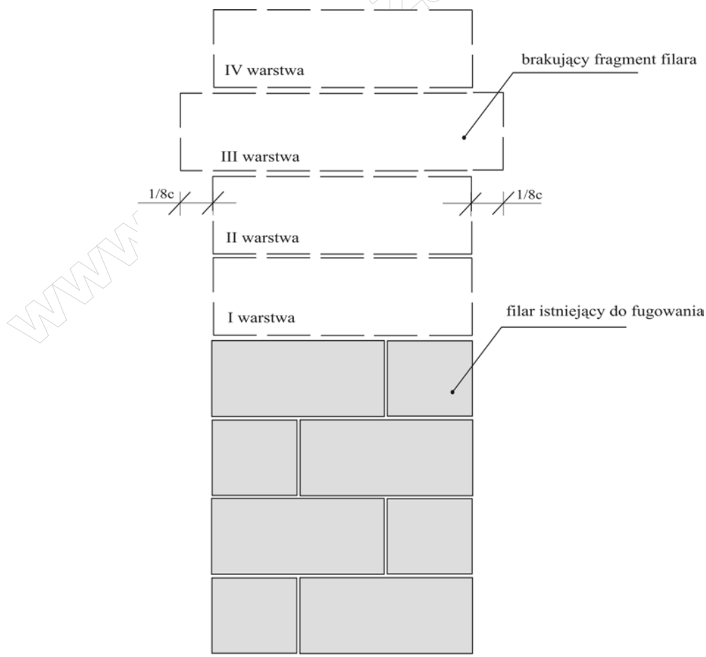
Rysunek 1. Widok filara (zaznaczona część do spoinowania i brakujące warstwy do wykonania)
