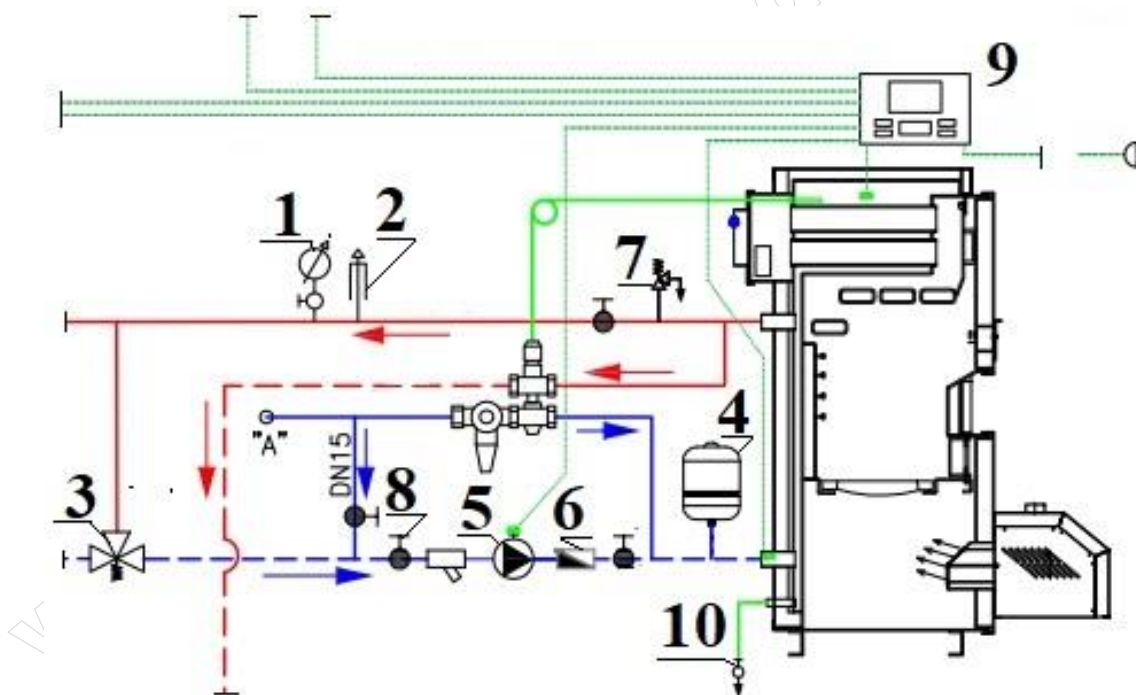
Rys. 1. Fragment instalacji kotła na biomasę
