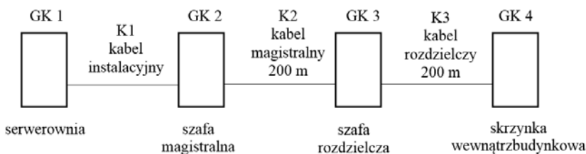
Rysunek 3. Schemat sieci telefonicznej
