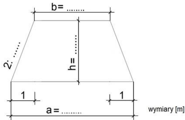
Rysunek 2. Przekrój poprzeczny pojedynczej przyzmy
