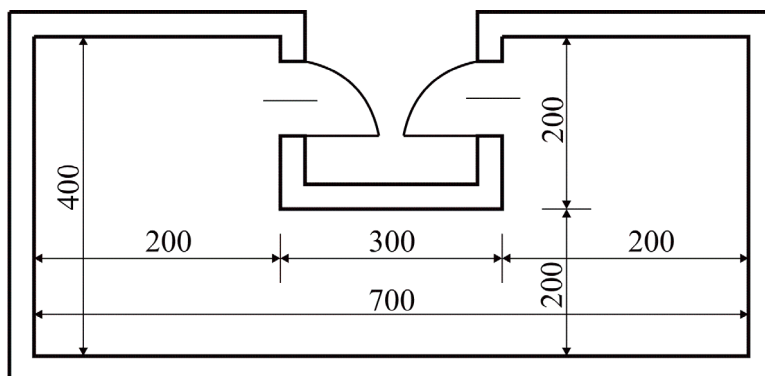
Rys. Rzut poziomy
