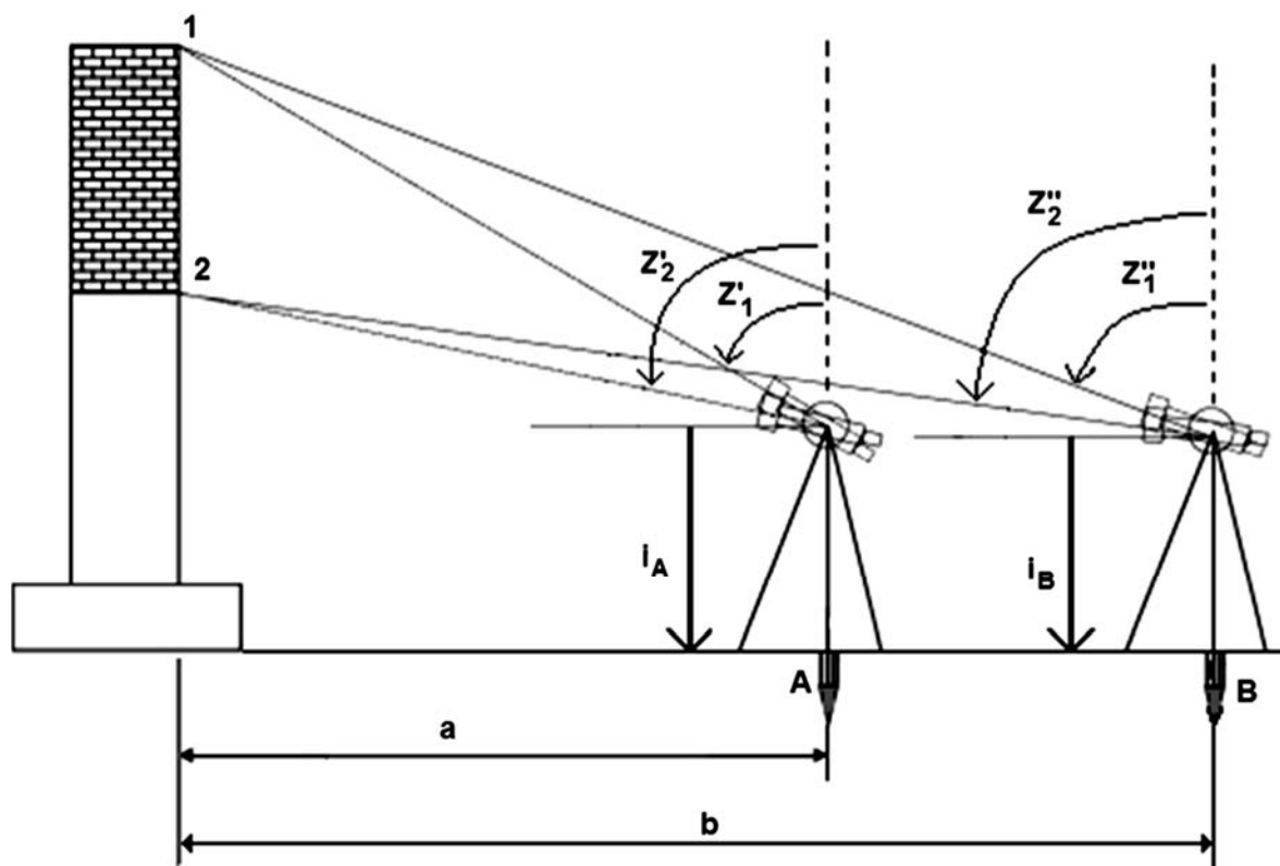
SZKIC SYTUACYJNY POŁOŻENIA PUNKTÓW
