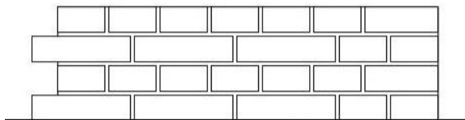
Rysunek 2. Widok A-A fragmentu lica muru
