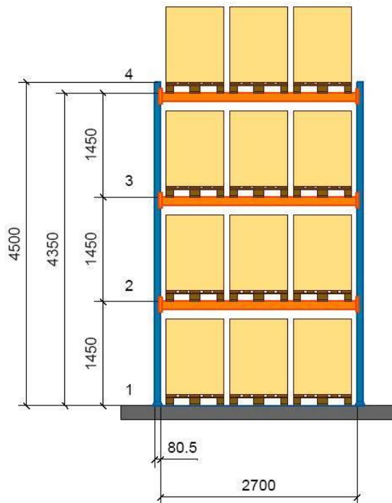
Ilustracja pogłówna ramowego regału magazynowego z wymiarami w mm
