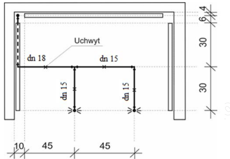
Rysunek 2. Rzut poziomy instalacji przeciwpożarowej, wymiary w centymetrach
