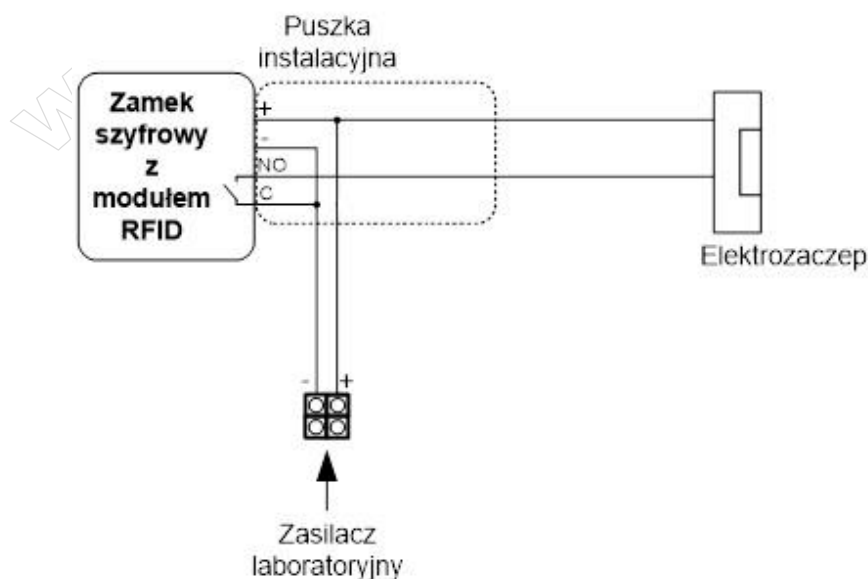
Rysunek 1. Schemat montażowy instalacji systemu kontroli dostępu
