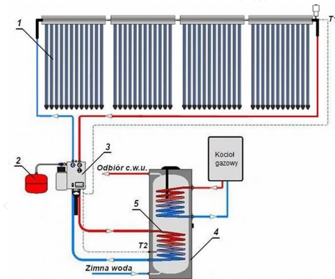
Rysunek 1. Schemat słonecznej instalacji grzewczej
