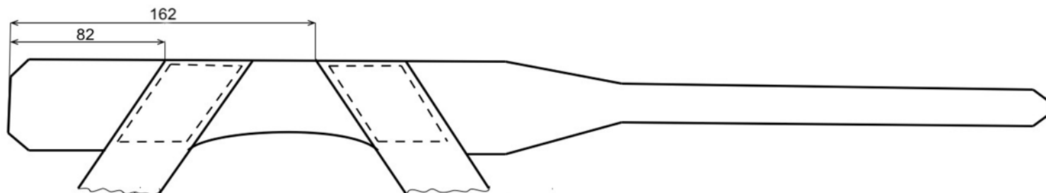
Rysunek 6. Naszytie na część główną paska nadkolanowego pasków łączących z lejem
