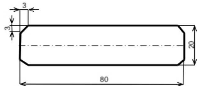
Rysunek 3. Szablon paska mocującego klamrę
