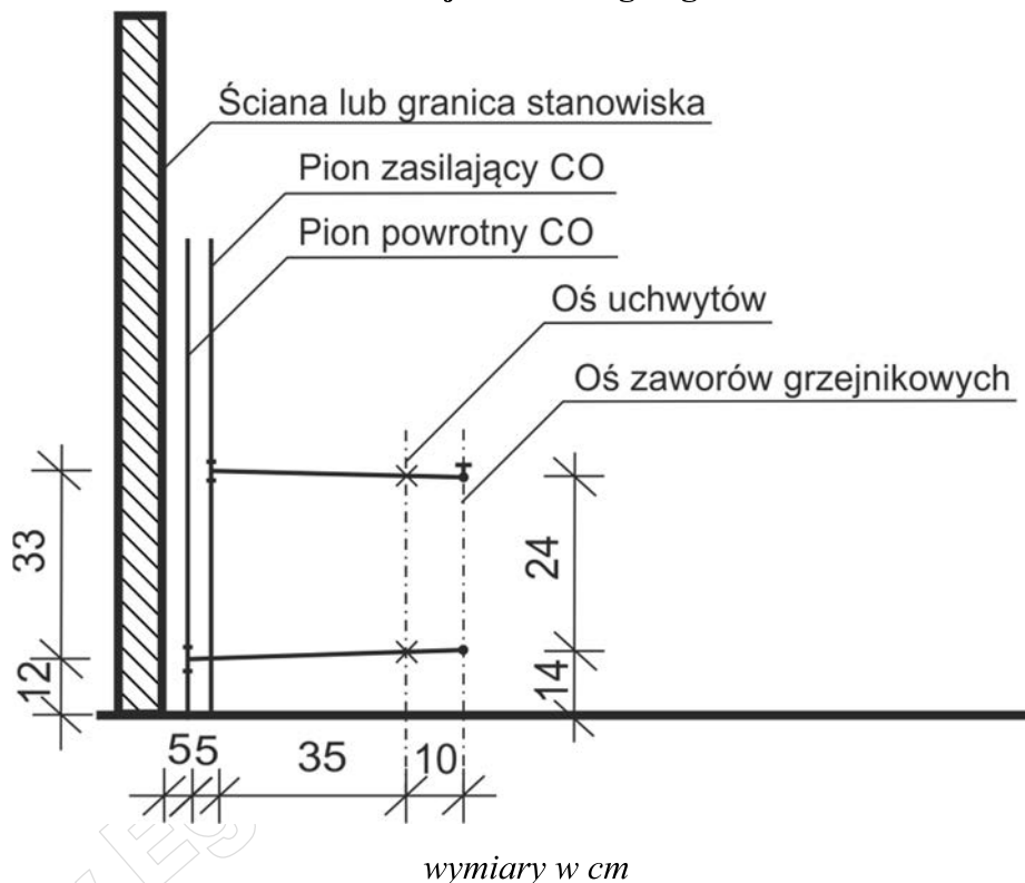
Widok instalacji centralnego ogrzewania
