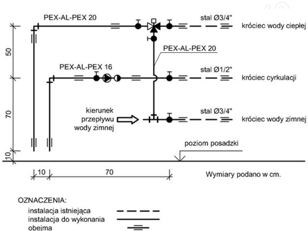
Rysunek 1. Podłączenie instalacji wody zimnej i ciepłej wody użytkowej do króćców zasobnika solarnego
