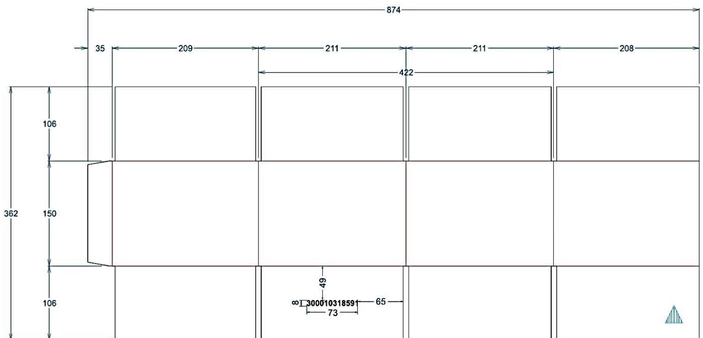
Rysunek 1. Konstrukcja i wymiary pudła
