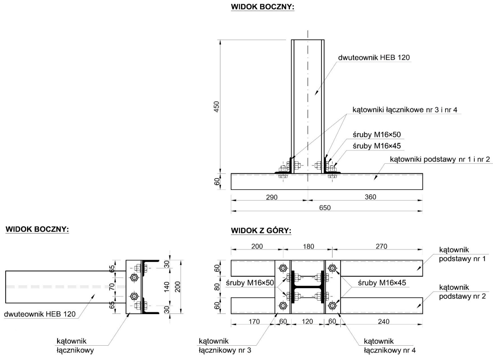
Rysunek 1. Rysunek zestawieniowy konstrukcji stalowej
