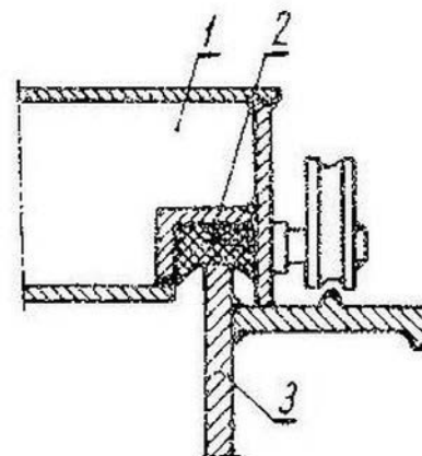
1-pokrywa 2-uszczelnienie gumowe 3- zrębica luku
