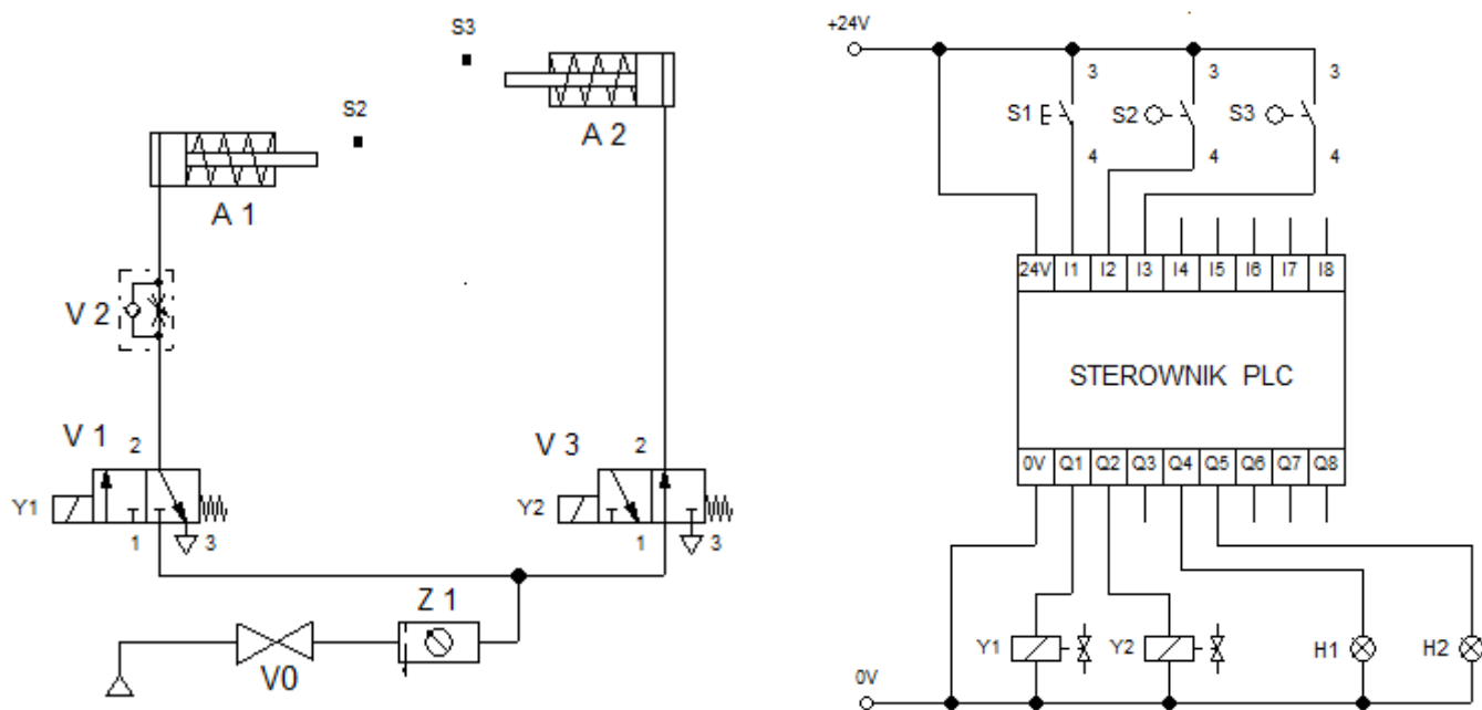
Rysunek 1. Schemat połączeń pneumatycznych i elektrycznych układu elektropneumatycznego, przygotowanego na stanowisku
