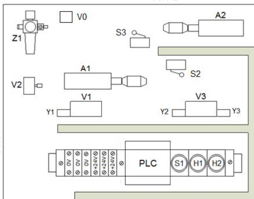
Rysunek 1. Schemat połączeń pneumatycznych i elektrycznych układu elektropneumatycznego, przygotowanego na stanowisku
