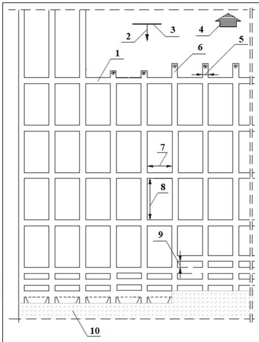
Rysunek 1. Schemat systemu komorowo-filarowego z podszadką hydrauliczną
