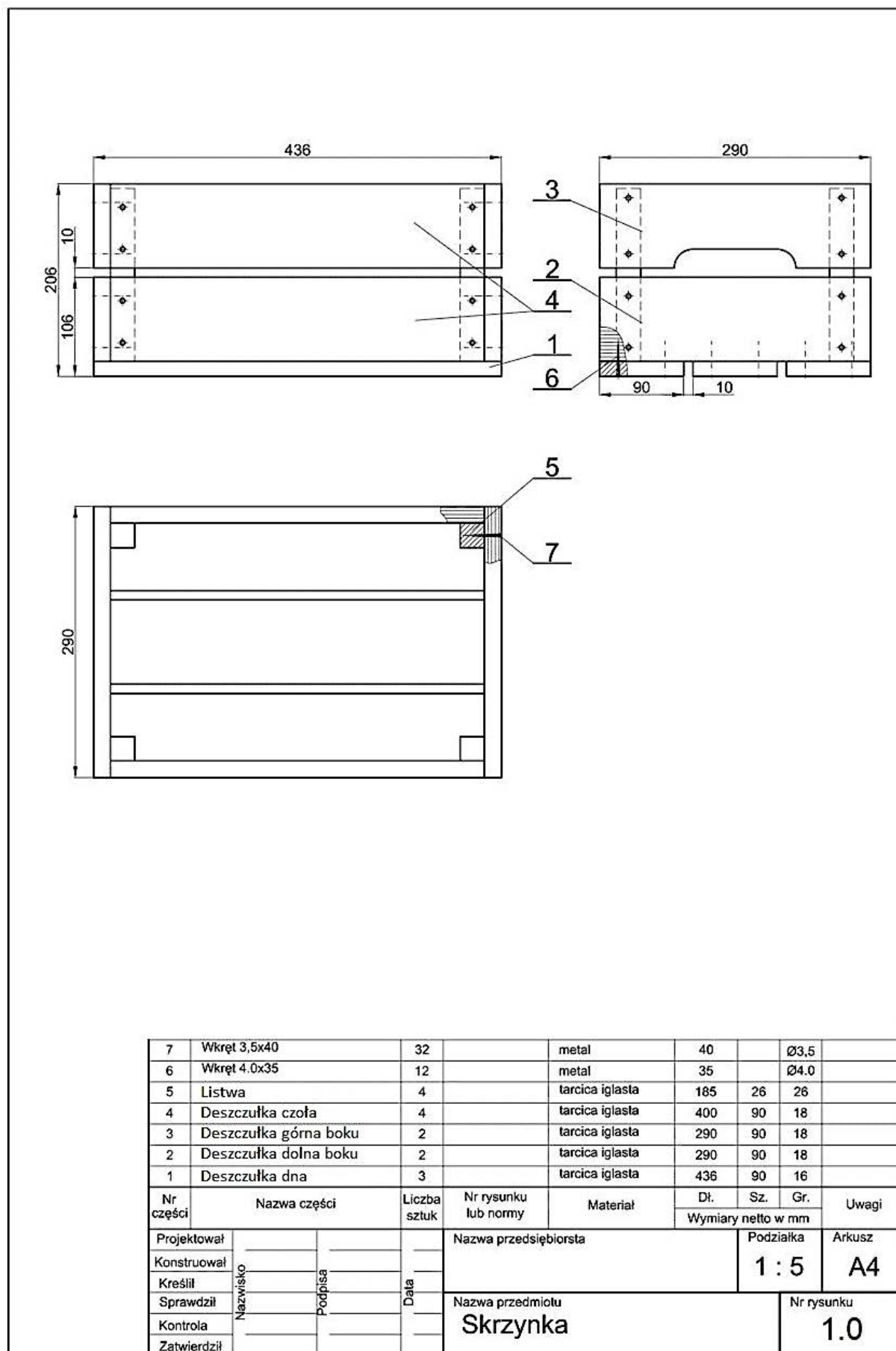
Rysunek 1. Rysunek złożeniowy skrzynki
