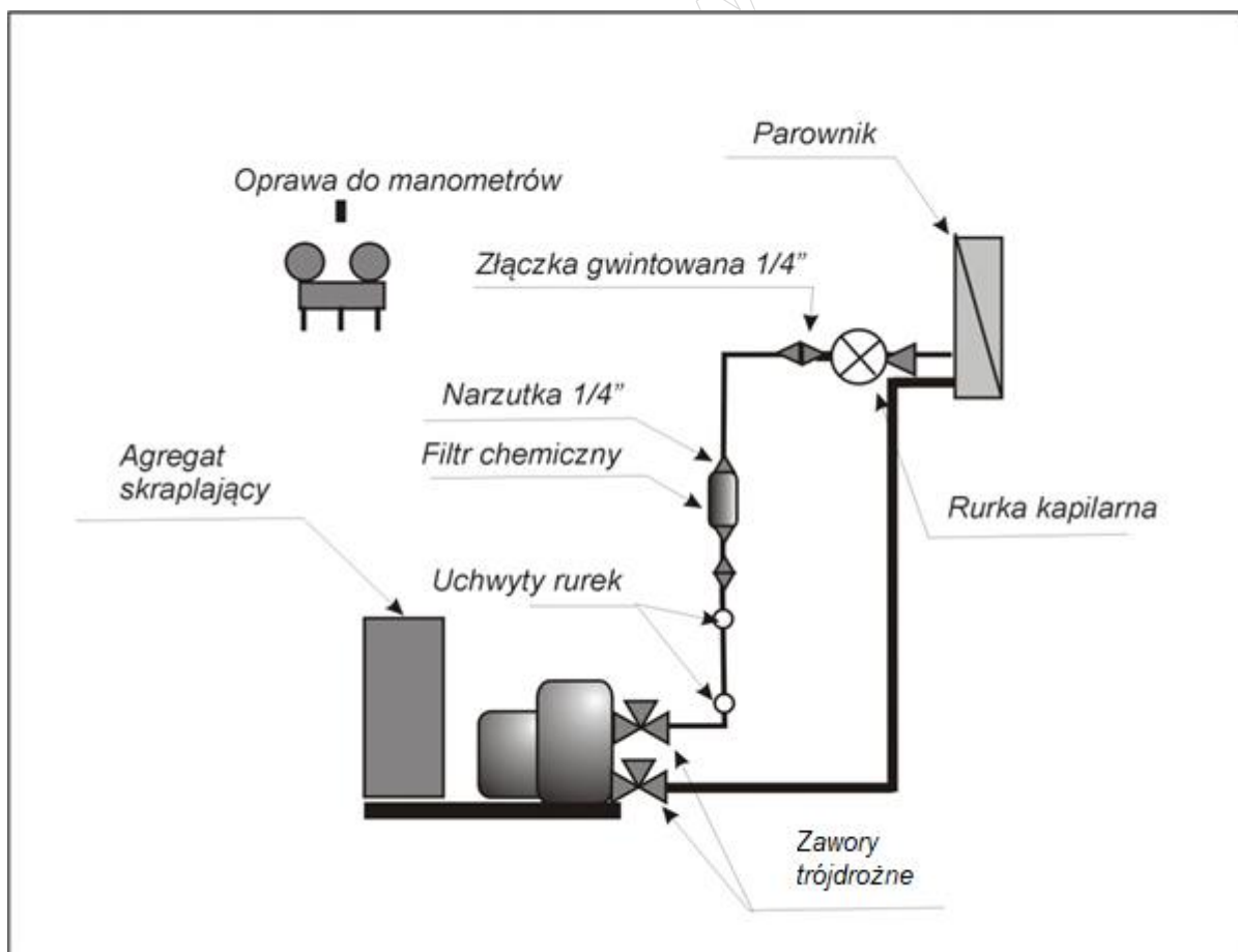
Rysunek 1. Schemat urządzenia chłodniczego
