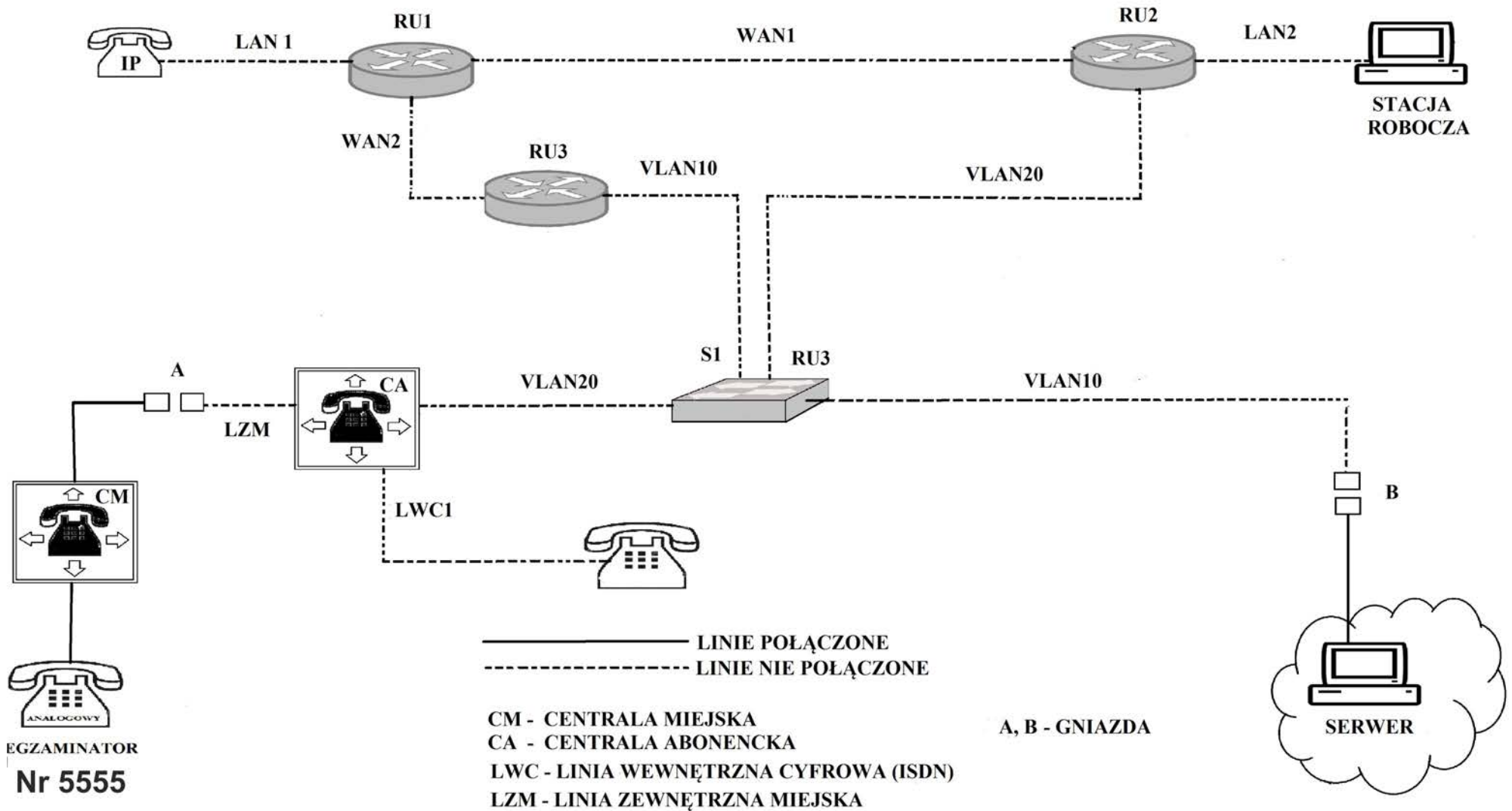
Schemat usytuowania urządzeń w sieci teleinformatycznej
