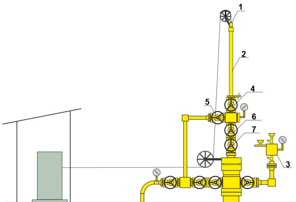
Rysunek 1. Wyposażenie napowierzchniowe odwiertu SX-7A
