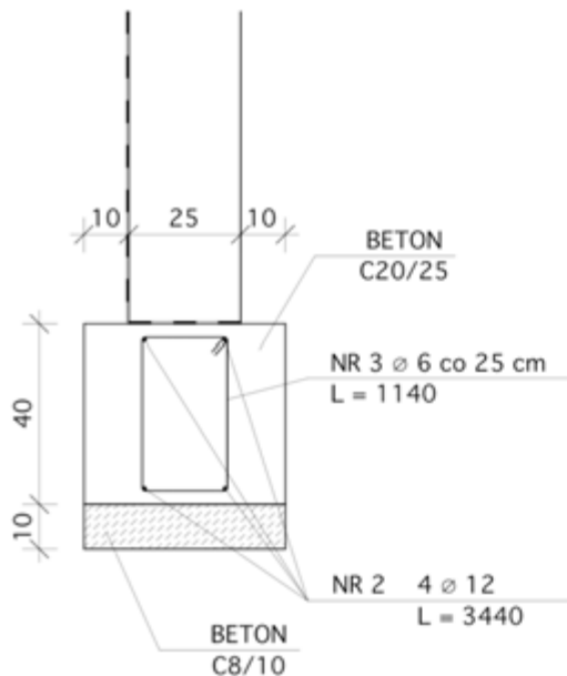
Ława fundamentowa Ł-1
