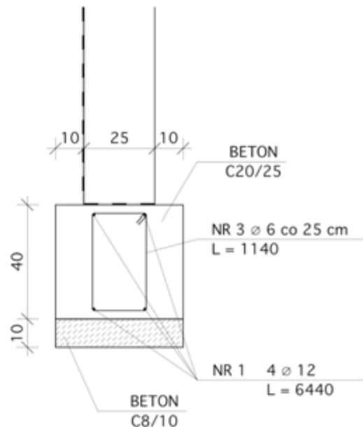
Ława fundamentowa Ł-2
