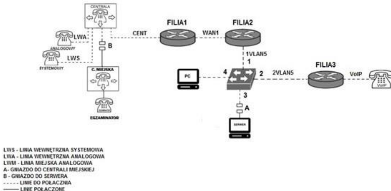
Schemat usytuowania urządzeń w sieci teleinformatycznej
