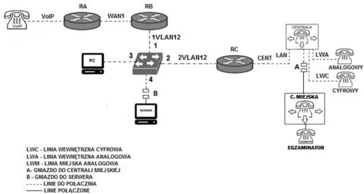
Schemat usytuowania urządzeń w sieci teleinformatycznej
