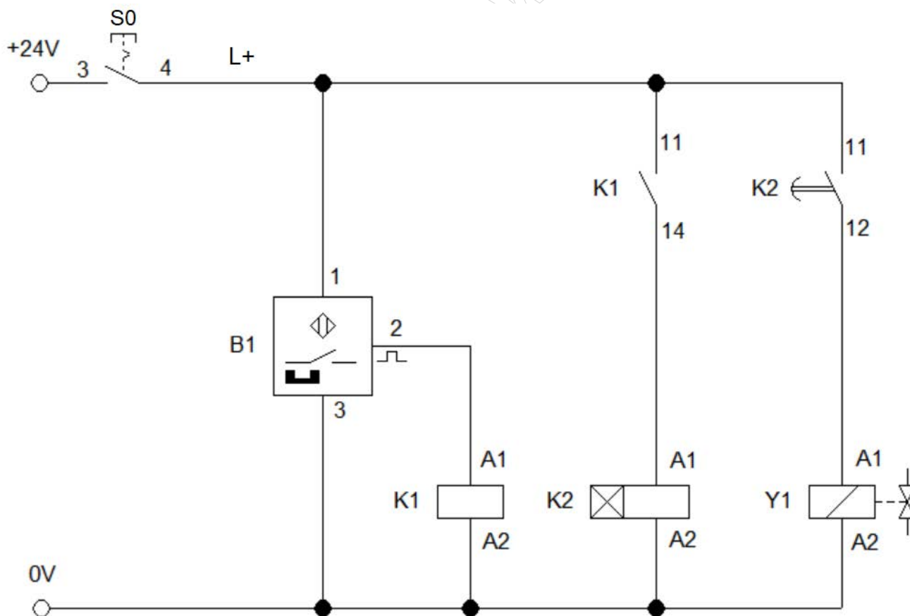
Rysunek 2. Schemat elektryczny układu elektropneumatycznego
