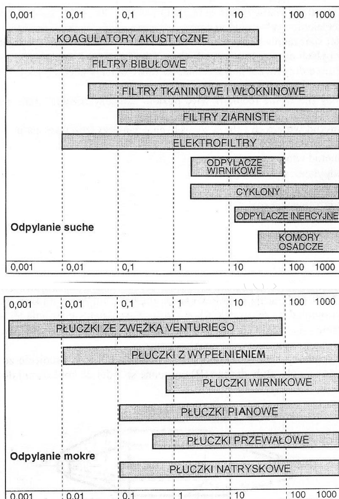
Rys. Rodzaje odpylaczy suchych i mokrych i ich zakres zdolności odpylania ziaren o określonej granulacji w μm
