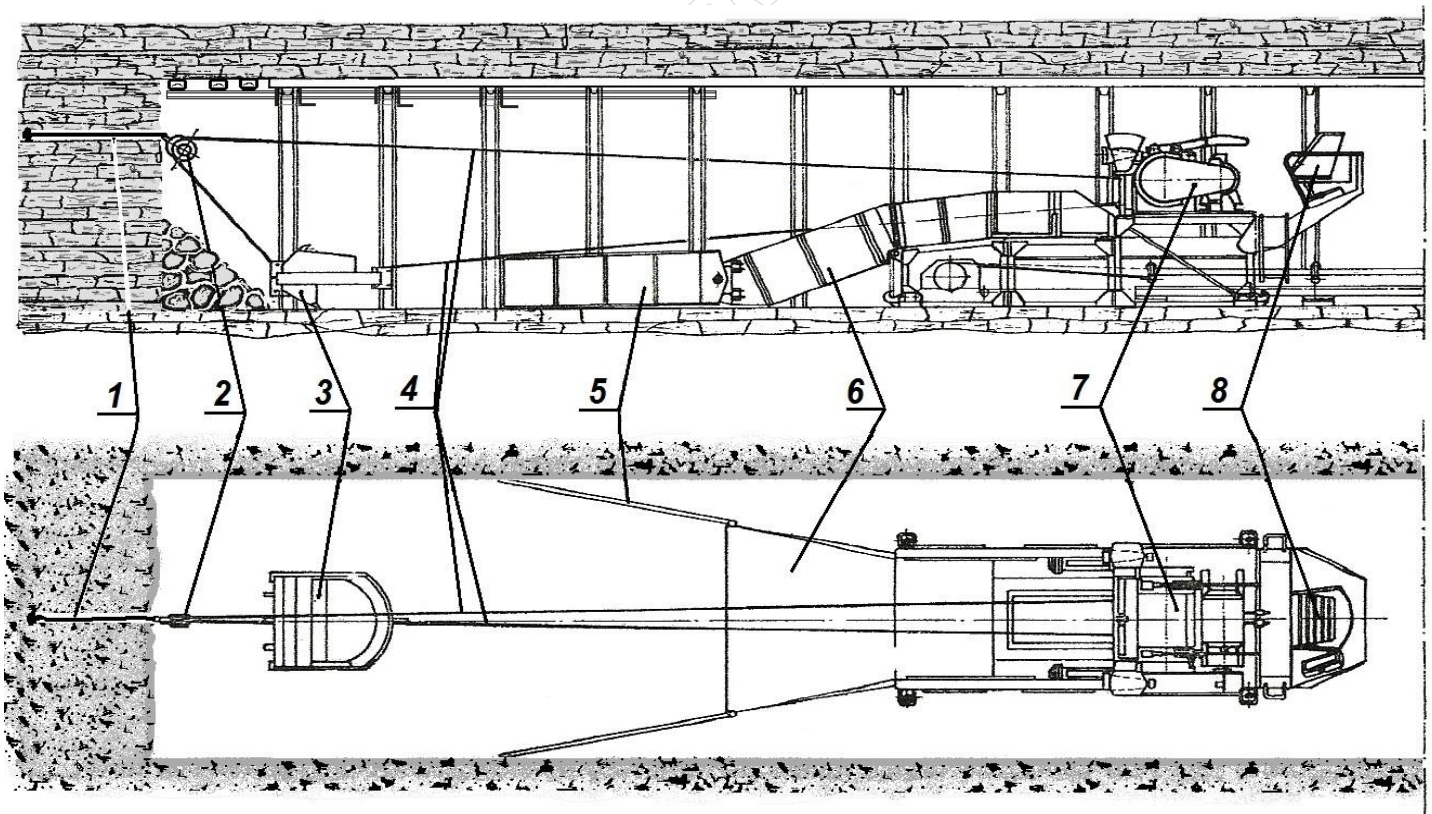
Rysunek 1. Wybrane elementy wyposażenia drążonego chodnika C-3
