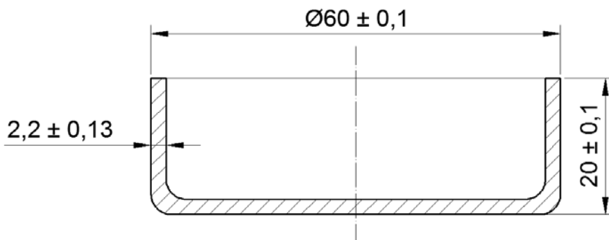
Główne wymiary wytłoczki
