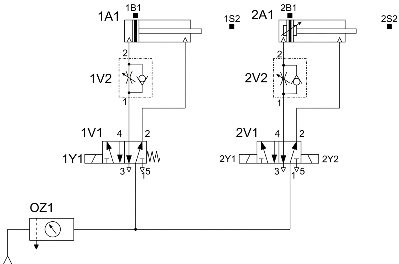
Rysunek 1. Schemat połączeń elementów pneumatycznych urządzenia mechatronicznego
