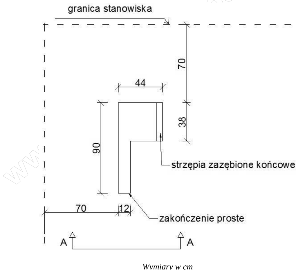
Rysunek 1. Rzut fragmentu narożnika do wymurowania
