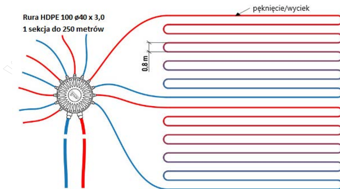
Rysunek 2. Schemat fragmentu wymiennika gruntowego meandrycznego z wskazanym miejscem uszkodzenia
