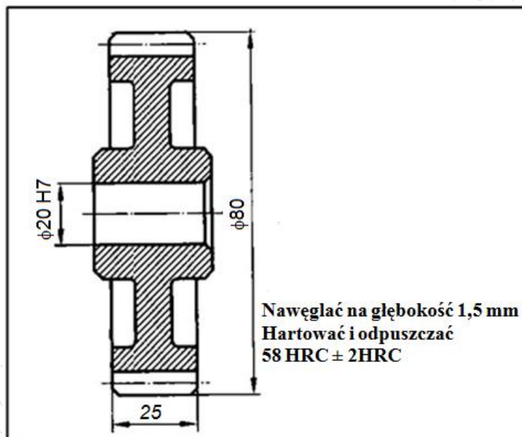
Rysunek 1. Główne wymiary i parametry obróbki cieplno-chemicznej koła zębatego walcowego o zębach prostych
