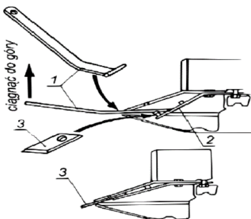
1- specjalny klucz, 2- trzymak nożyka, 3- nożyk
