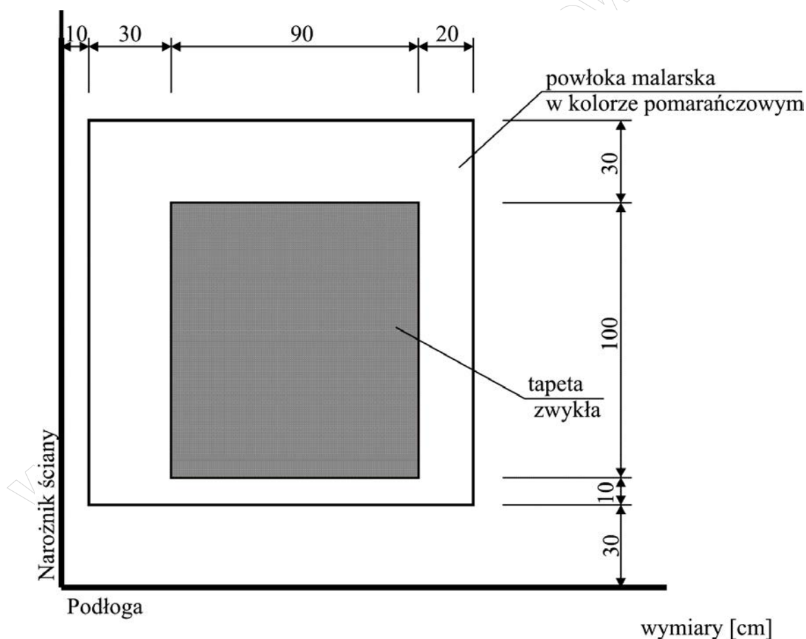
Rys. Widok fragmentu ściany przeznaczonej do malowania i tapetowania
