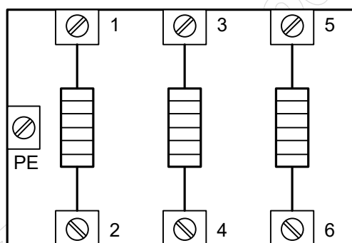
Rysunek 6. Moduł grzewczy
