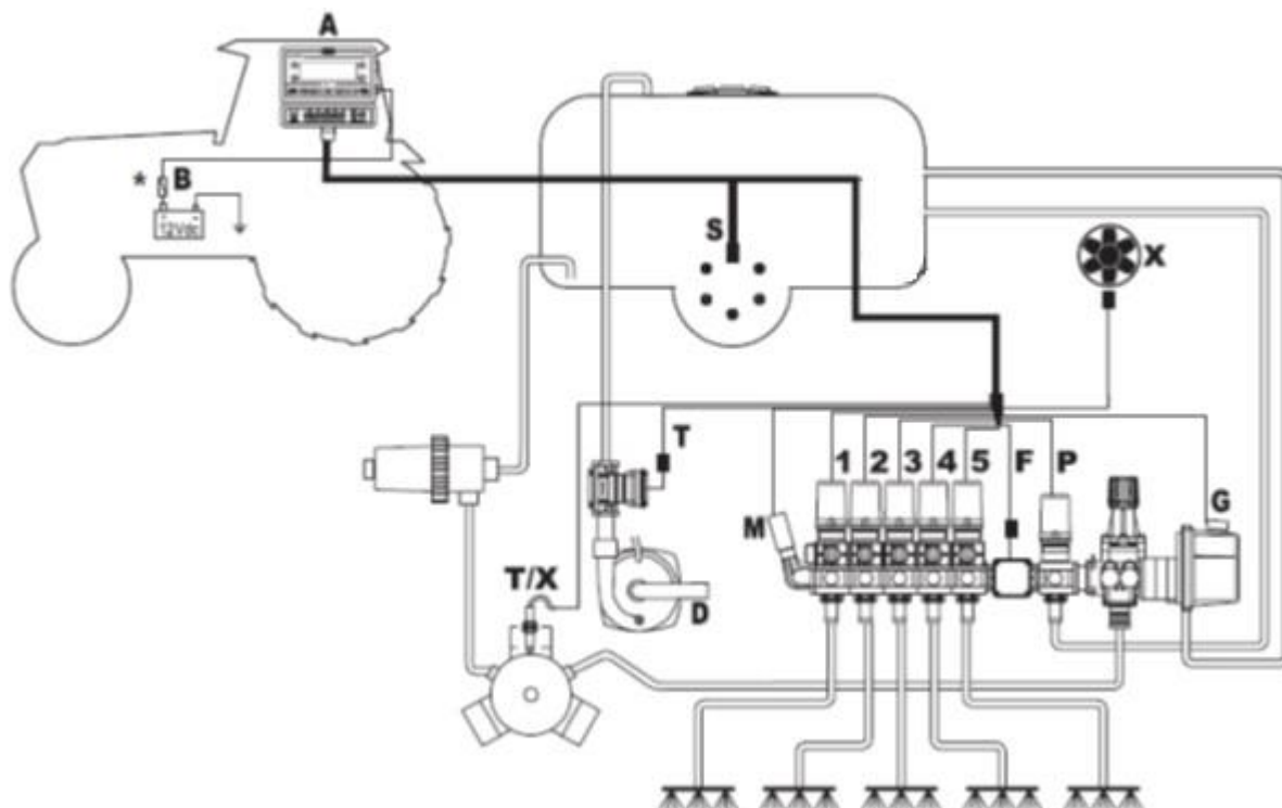
Rysunek 1. Schemat instalacji opryskiwacza
