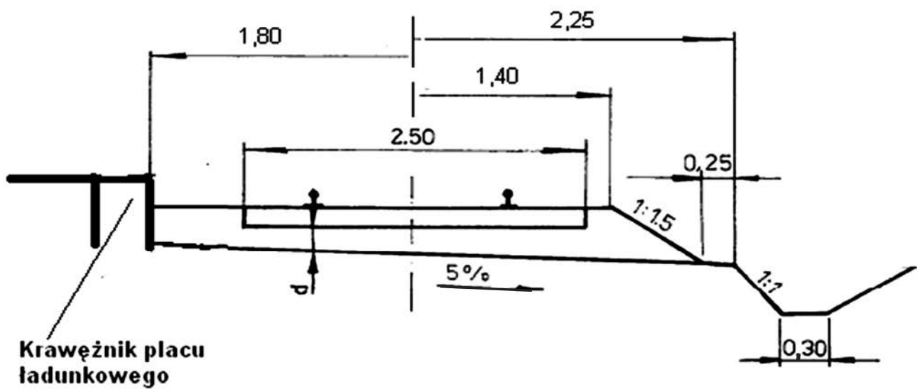
Rysunek 2. Przekrój poprzeczny nawierzchni i podtorza toru
