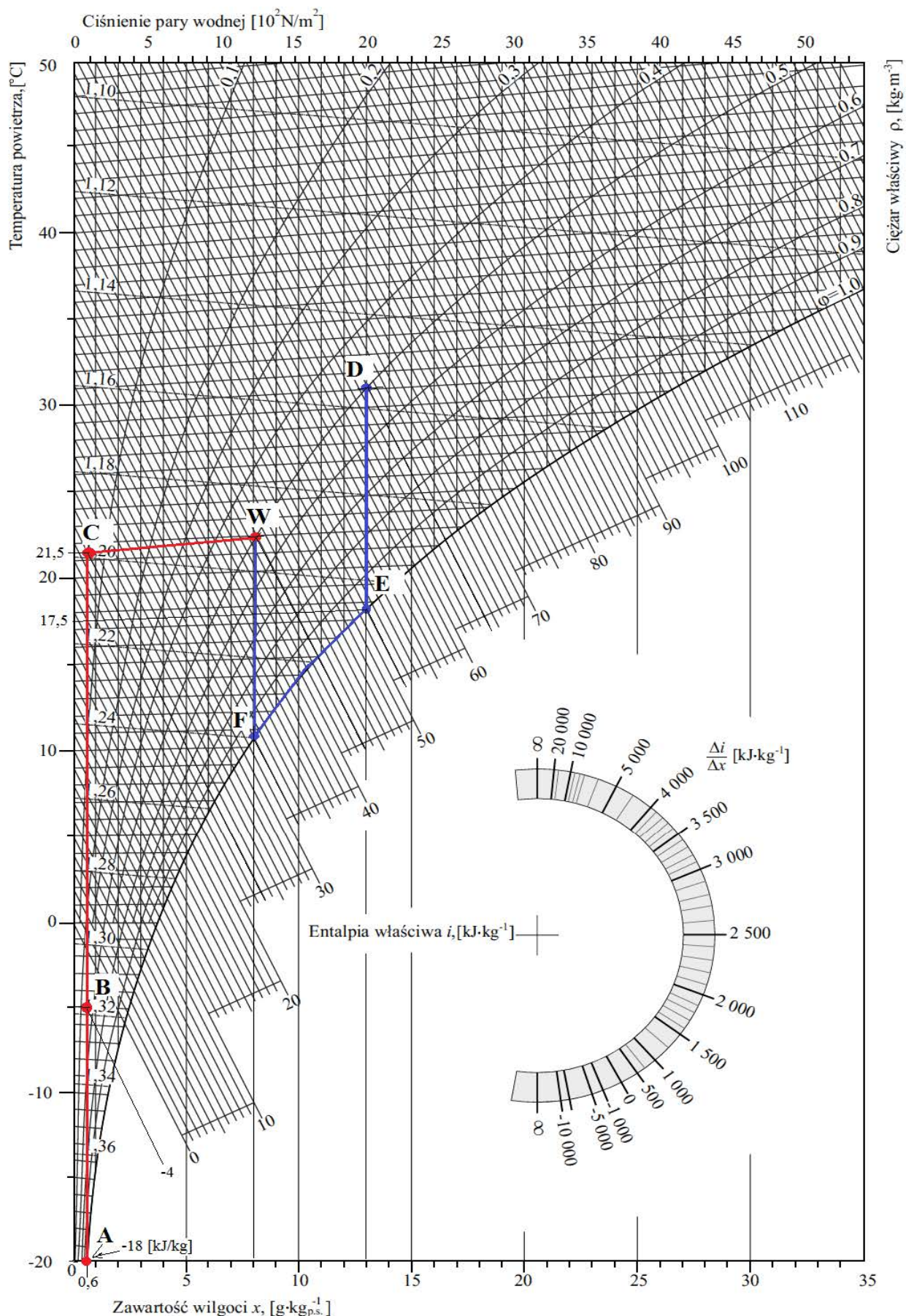
Rysunek 2. Obróbka ciepno-wilgotnościowa powietrza realizowana przez instalację klimatyzacyjną w okresie zimowym i letnim przedstawiona na wykresie Molliera
