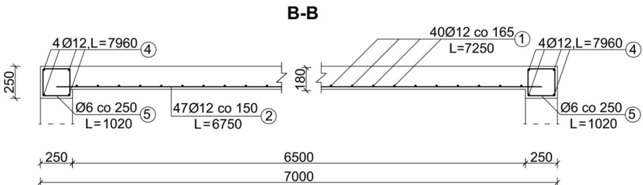
Rysunek konstrukcyjny żelbetowego stropu płytowego i wieńców stropowych – rzut i przekroje
