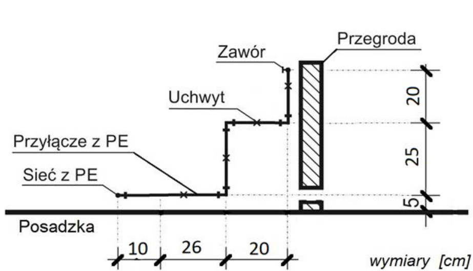
Rysunek 1. Przekrój pionowy przyłącza wodociągowego
