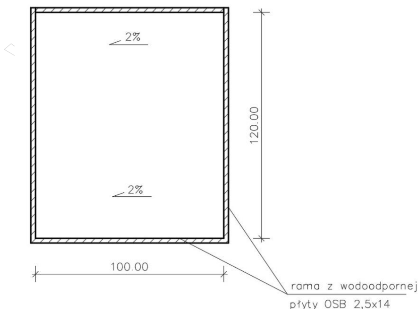
Rysunek.1 Rzut poziomy koryta pod warstwę odsączającą
