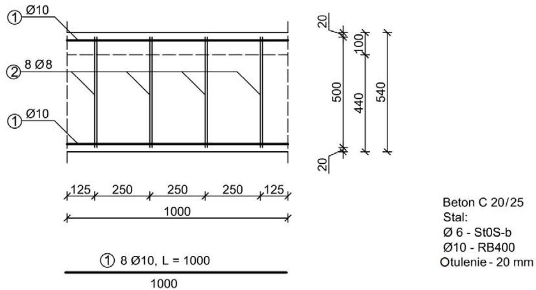
Rysunek konstrukcyjny zbrojenia belki żelbetowej
