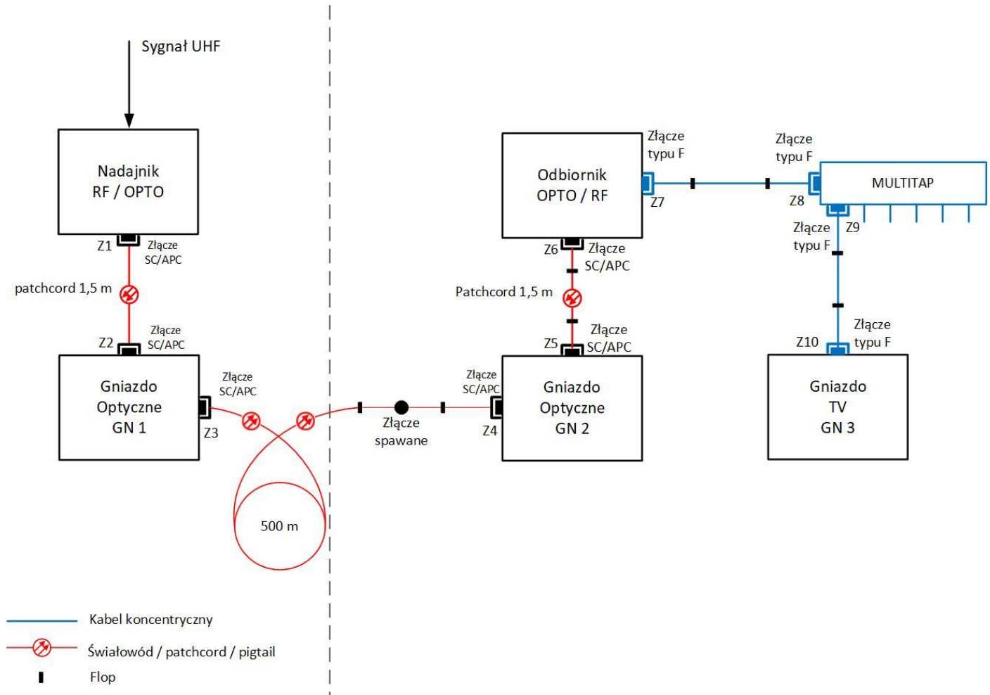
Rysunek 1. Schemat rozmieszczenia elementów instalacji na płycie montażowej
