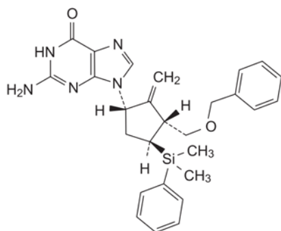
F. 2-amino-9-[(1S,3R,4S)-3-[(benzyloksy)metylo]-4-[dimetylo(fenilo)sililo]-2-metylidencyklopentylo]-1,9-dihydro-6H-puryn-6-on.
