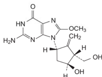
E. 2-amino-9-[(1S,3R,4S)-4-hydroksy-3-(hydroksymetylo)-2-metylidencyklopentylo]-8-metoksy-1,9-dihydro-6H-puryn-6-on,
