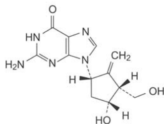
D. 2-amino-9-[(1S,3R,4R)-4-hydroksy-3-(hydroksymetylo)-2-metylidencyklopentylo]-1,9-dihydro-6H-puryn-6-on,
